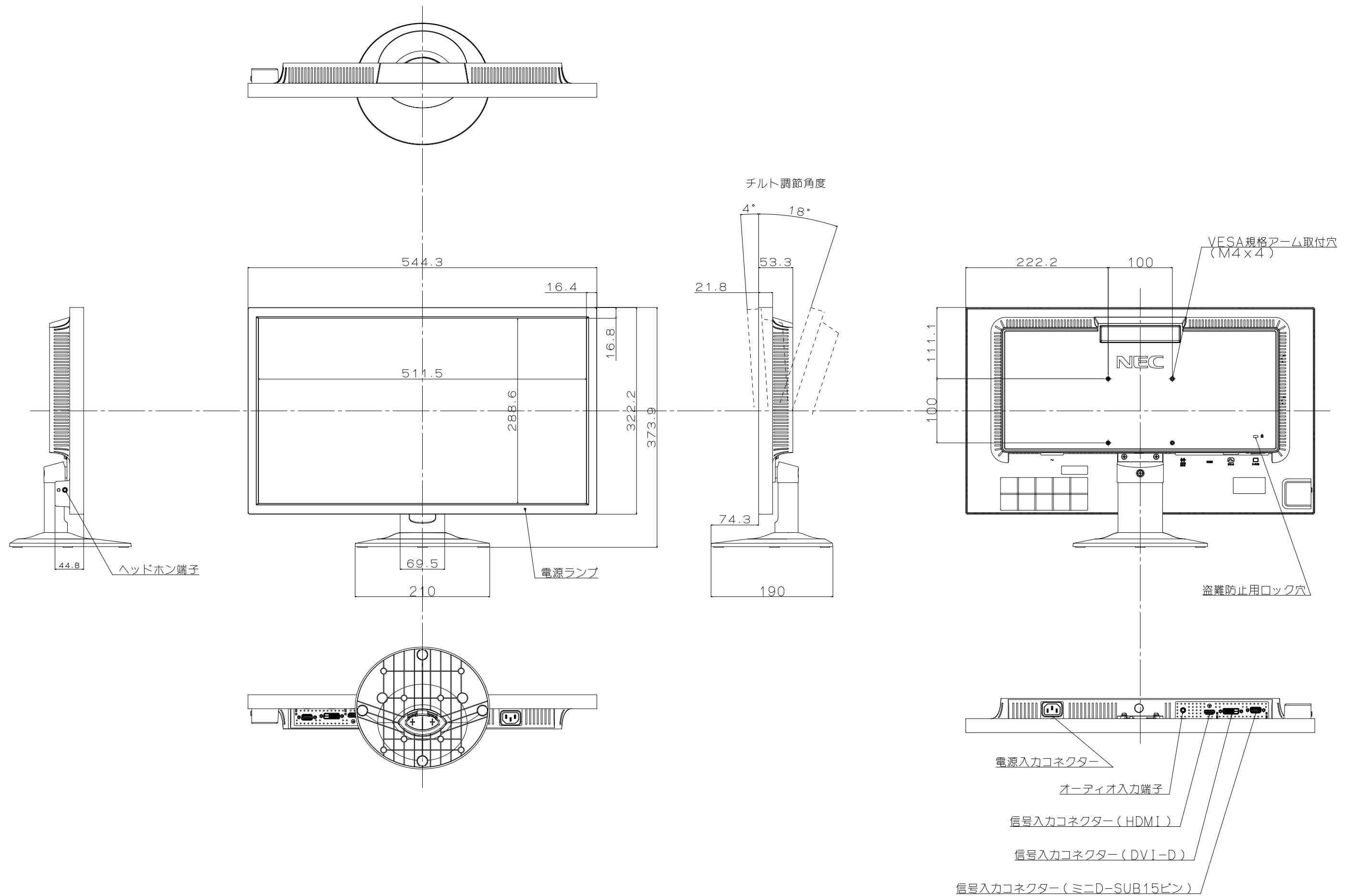
LCD-AS233WM-W5 外形図
