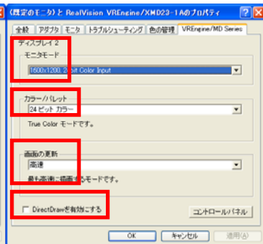
図 5.3-4 詳細設定
