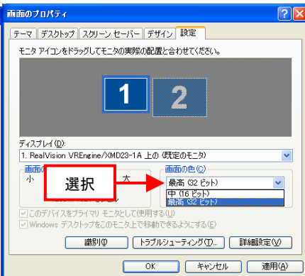
図 5.2-2 画面の色
