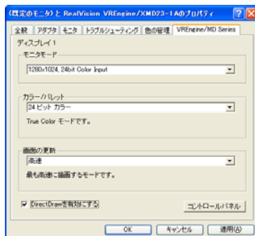
図 5.3-8 DirectDraw の設定
