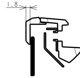
SECTION V0-V0 SCALE 1:1
