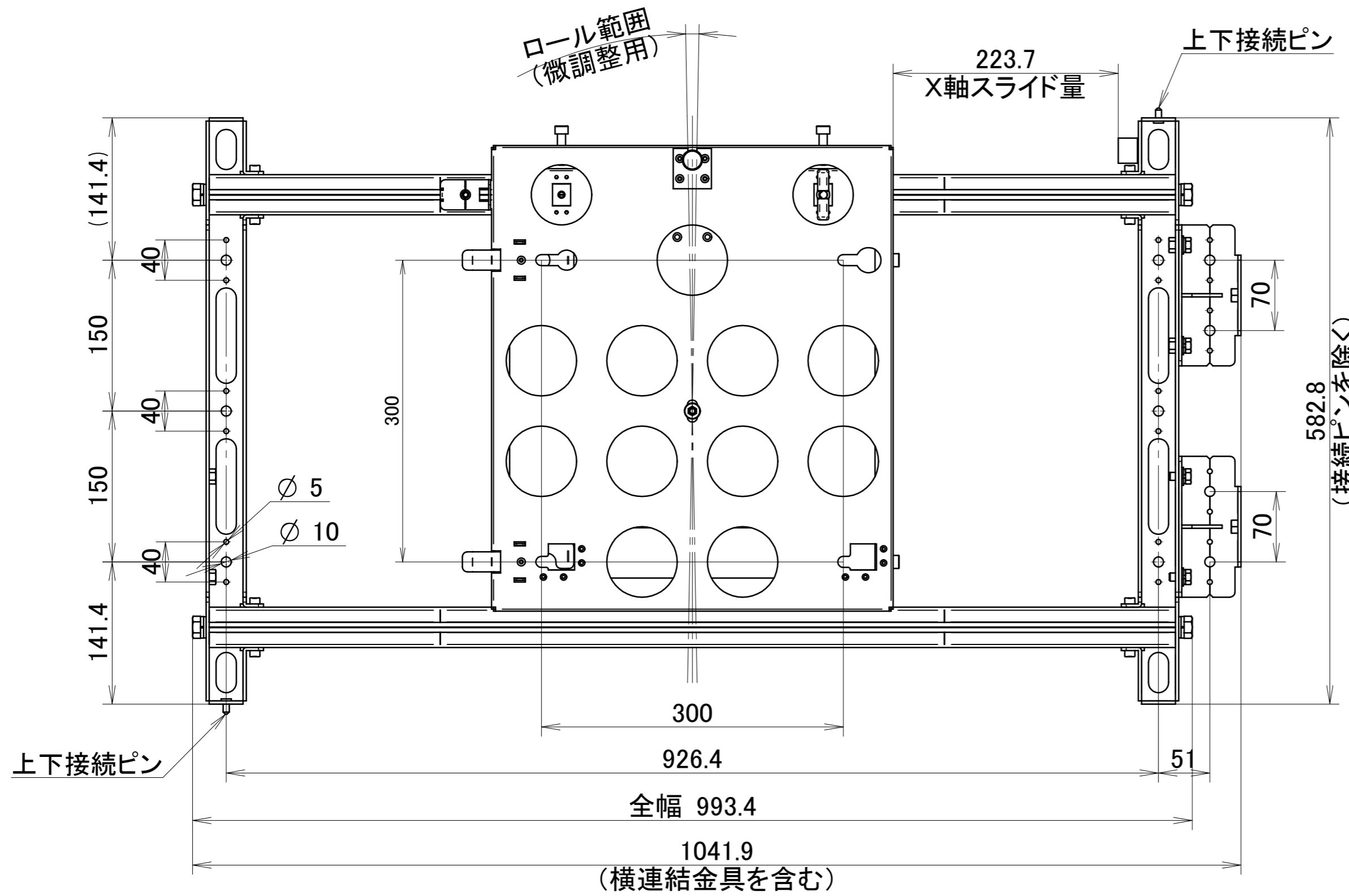
正面図
