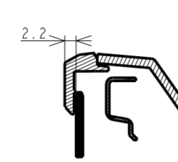
SECTION V0-V0 SCALE 1:1
