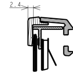
SECTION V0-V0 SCALE 1:1
