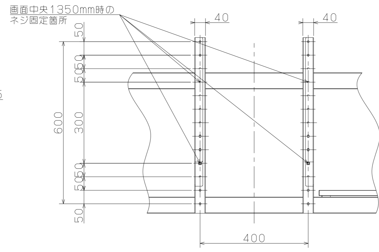
A部詳細(1:8)
